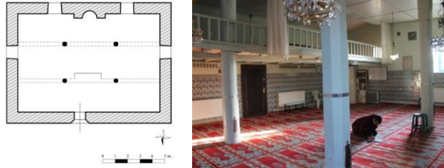
Çiz. 13, Foto. 38: Esenkent Köyü Camii planı ve harimi
