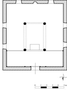
Çiz. 5, Foto. 13: Azat Köyü Camii planı ve genel görünümü
