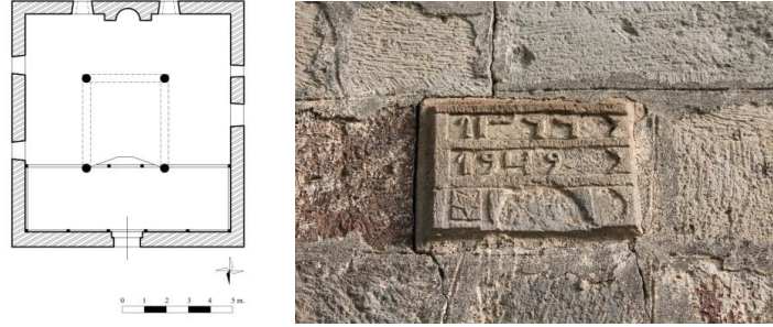
Çiz. 18, Foto. 49: Karakale Köyü Camii planı ve kitabesi
