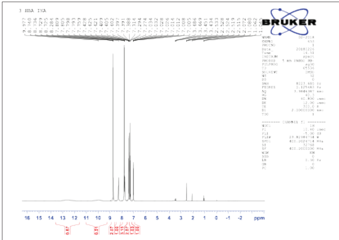
Şekil 2. Ko-kristalin ^1\text{H} NMR spektrumu.
