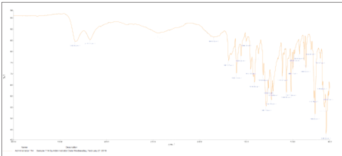
Şekil 6. Ko-kristal molekülünün FT- IR spektrumu.
