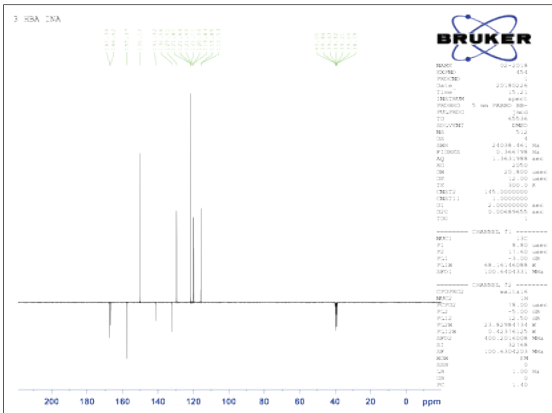
Şekil 3. Ko-kristalin ^{13}\text{C} NMR spektrumu.
