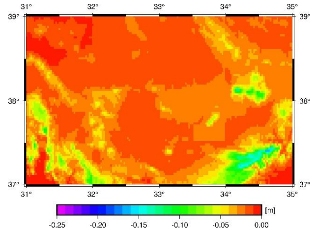
Şekil 5. Sabit yoğunluk modeli ve EPCRUSt modeli ile belirlenen jeoit yüksekliklerinin farklarının dağılımı
